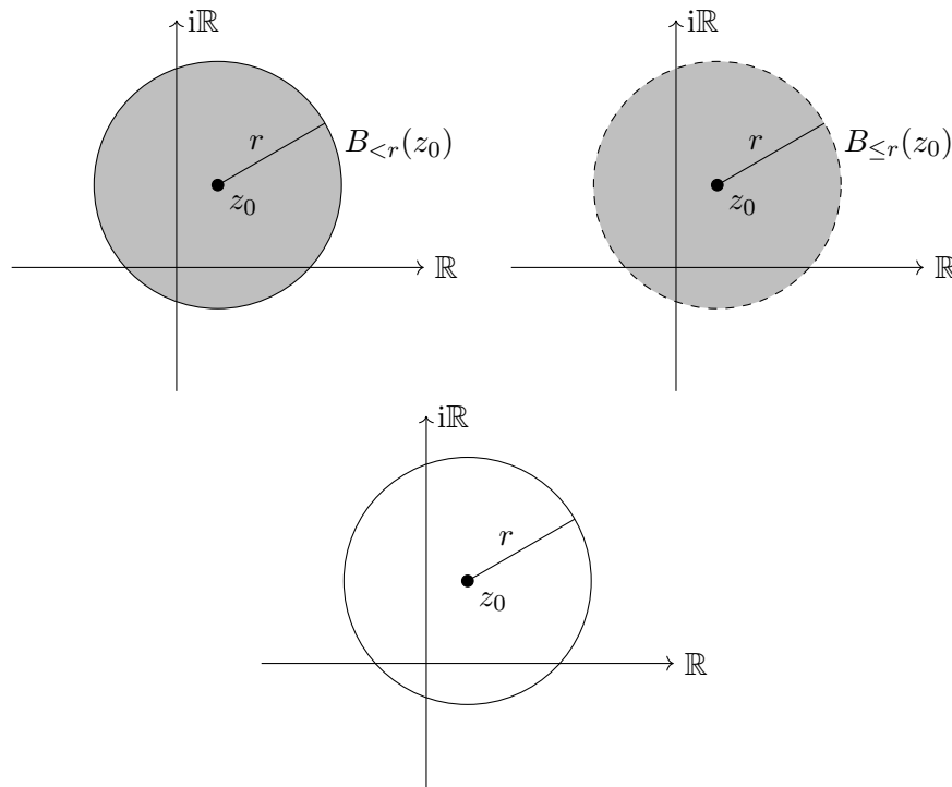
Abbildung 1.3.1: Skizzen der drei Mengen aus Beispiel 1.3.6: Die offene Kreisscheibe B_{<r}(z_0) , die abgeschlossene Kreisscheibe B_{\leq r}(z_0) und die Kreislinie mit Mittelpunkt z_0 und Radius r .
